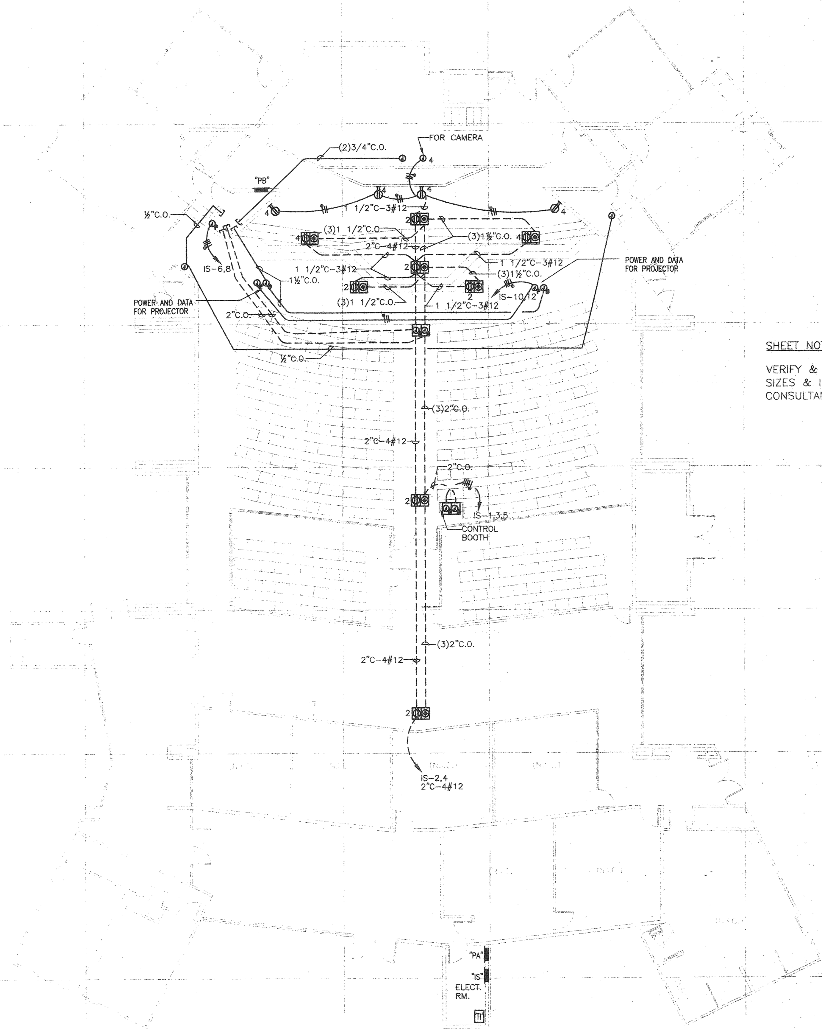
POWER PLAN SCALE: 1/8"=1'-0"
